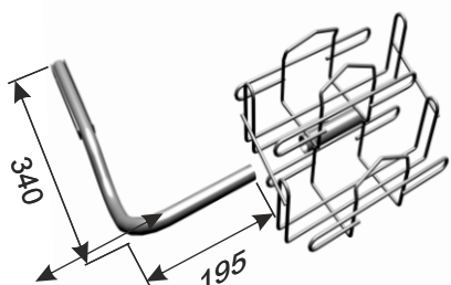
Left grip
