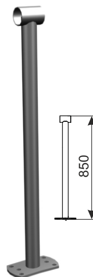
5. Middle pipe bumper module „foot”
