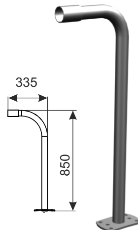
3. Side pipe bumper module „foot”
