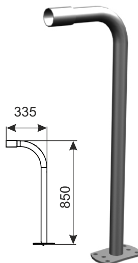
4. Side pipe bumper module „foot”
